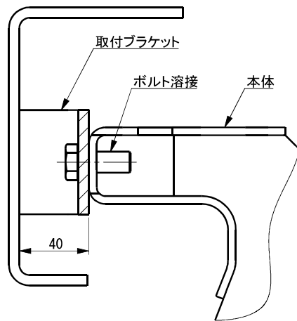
図1 現行本体取付
