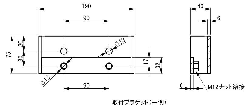
取付ブラケット(一例)
