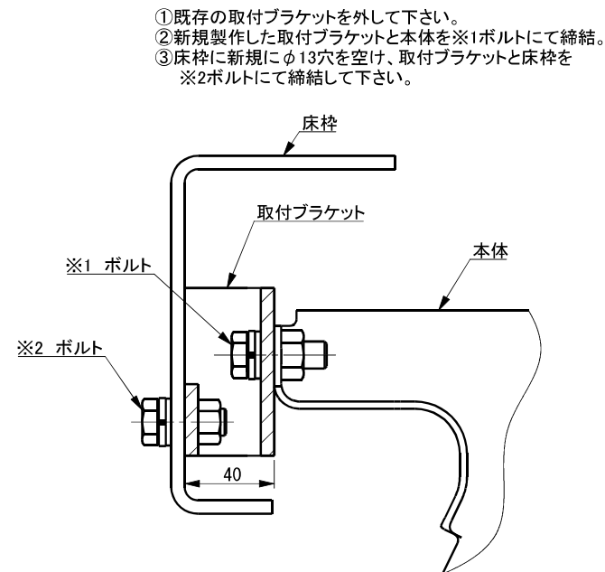
図2 新本体取付案(参考)
