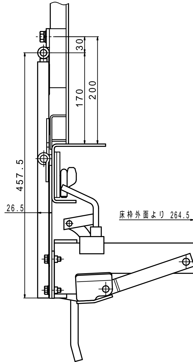
名称 セイコークットII型 - M(単車用) 外観図
